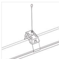
Suspensão com cabos (versão ROOF)
