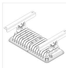
Suspensa giratória regulável
