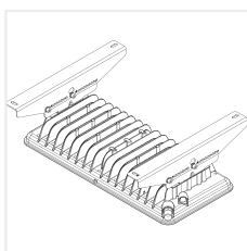
Suspensa giratória extraível
