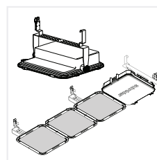
BASE, COMBI & MODULE Fixação com gancho
