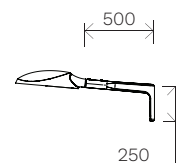
CONSOLA MURAL BRAÇO TRASEIRO
